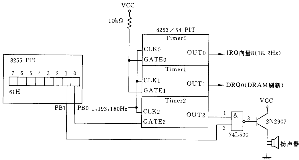
图 10.9 扬声器驱动系统
