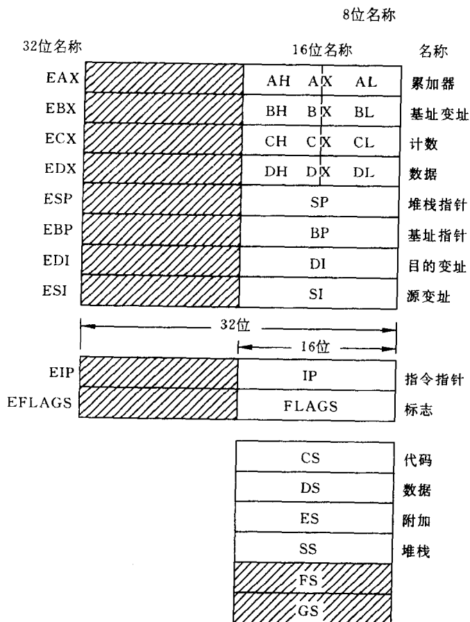
图 2.3 80x86 的程序可见寄存器组
