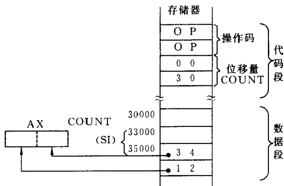
图 3.5 例 3.9 的执行情况
