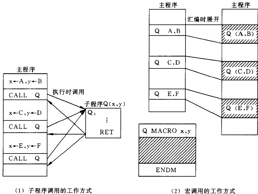
图 7.1 子程序调用和宏调用工作方式的区别
