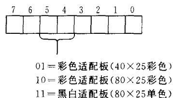
图 10.1 设备标志字
