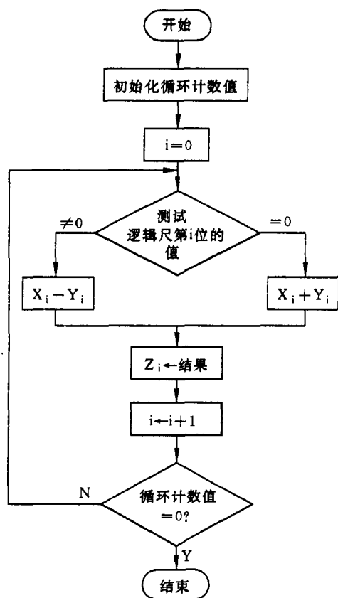
图 5.6 例 5.5 的程序框图
