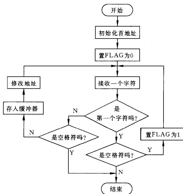
图 5.7 例 5.6 的程序框图
