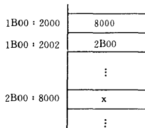
图 3.29 3.14 题的存储区情况
