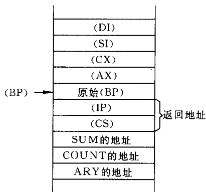
图 6.2 例 6.4 用堆栈传送参数地址时,堆栈最满时的状态
