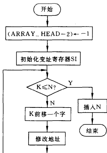
图 5.5 数组中插入一元素的程序框图
