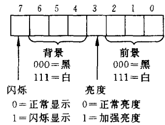
图 9.5 单色显示的属性字节
