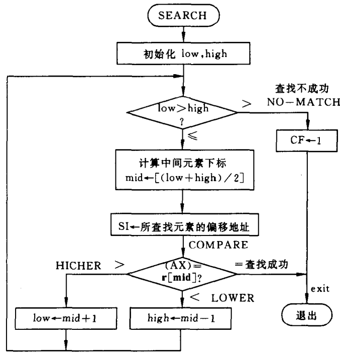
图 5.11 折半查找算法的程序框图
