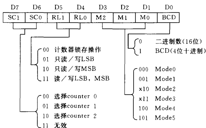
图 10.8 8253/54 的控制字格式
