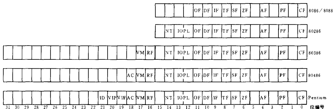
图 2.4 80x86 的标志寄存器
