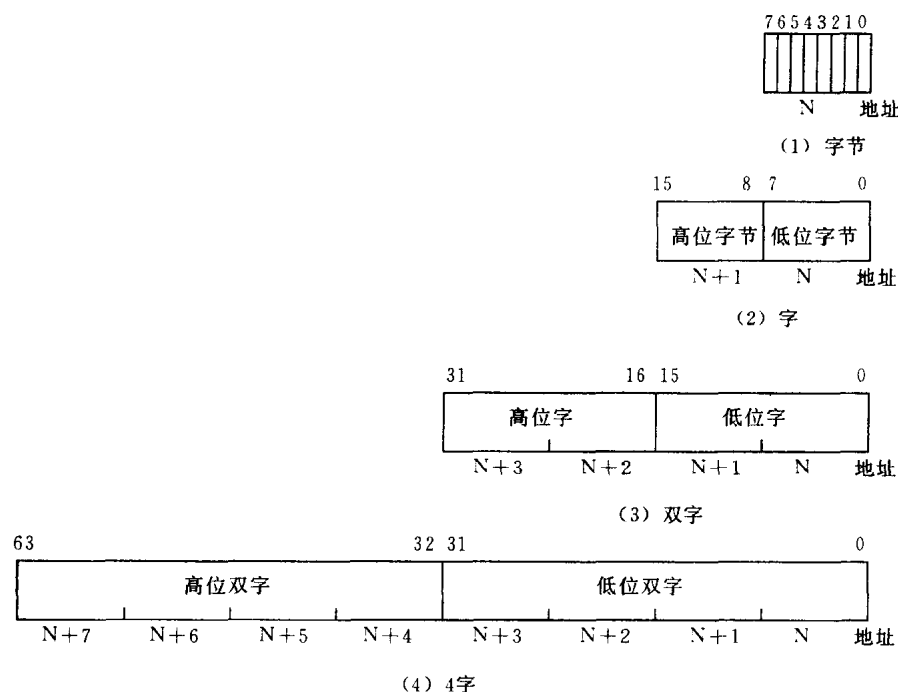
图 2.5 数据类型
