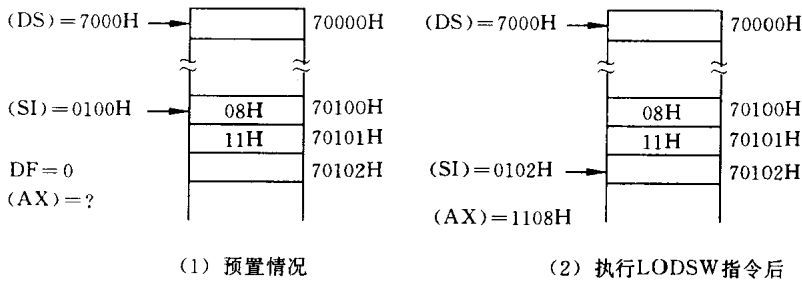
图 3.18 LODSW 指令的执行情况
