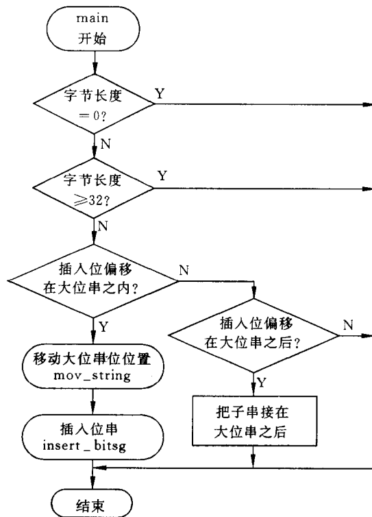
(1) 主程序框图
