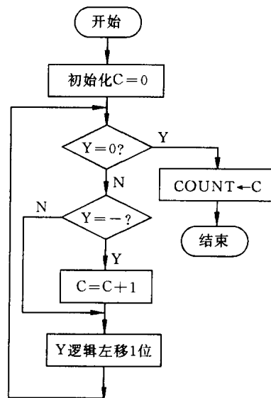
图 5.3 数 1 的程序框图
