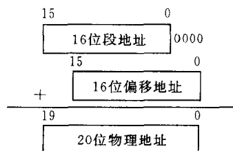
图 2.7 实模式存储器寻址时物理地址的计算方法
