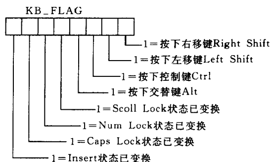
图 9.2 键盘状态字节
