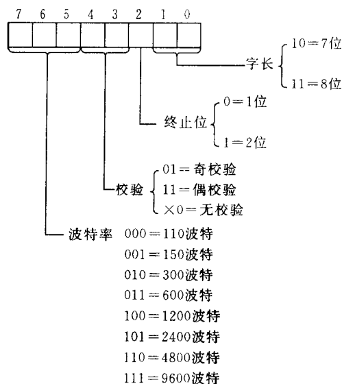
图 9.12 串行通信口初始化参数
