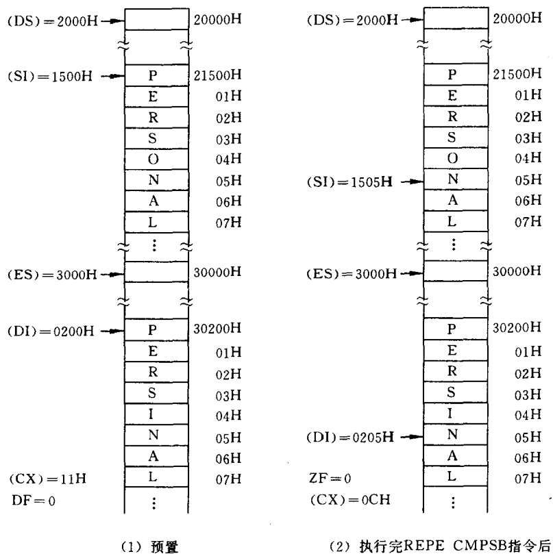
图 3.20 REPE CMPSB 指令的执行情况
