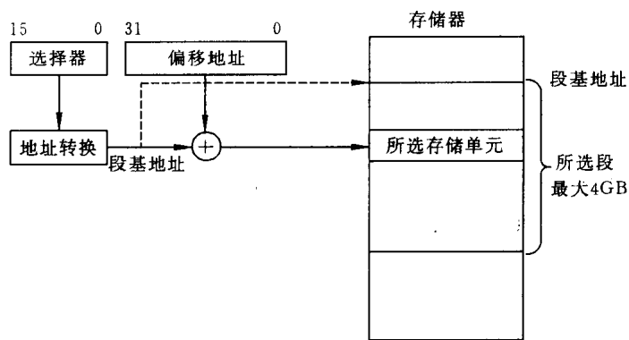
图 2.11 保护模式存储器寻址示意图
