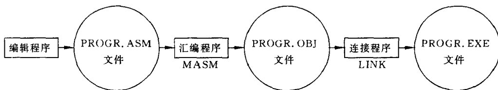
图 4.1 汇编语言程序的建立及汇编过程
