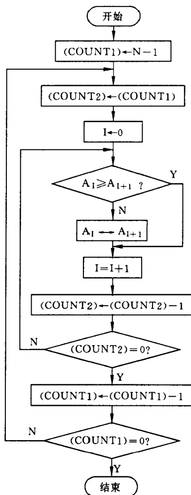
图 5.8 例 5.7 起泡排序算法的程序框图
