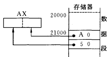
图 3.4 例 3.7 的执行情况
