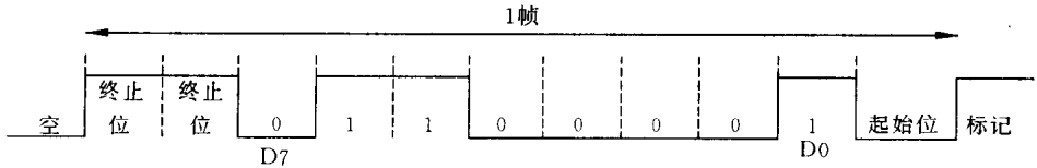
图 9.10 组帧后的 ASCII“a”(61H)
