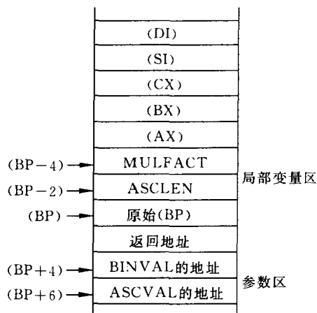
图 6.4 例 6.8 程序运行过程中堆栈最满时的状态
