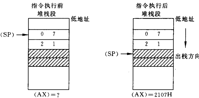
图 3.11 POP AX 指令的执行情况
