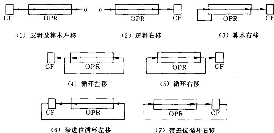
图 3.14 移位指令的操作
