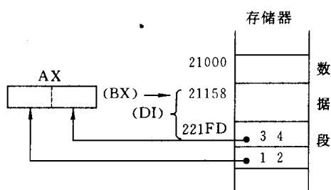
图 3.6 例 3.10 的执行情况
