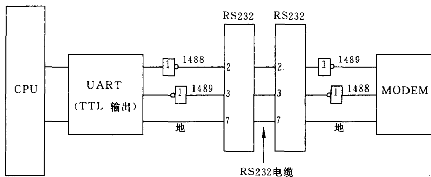
图 9.11 UART 与 RS232 的连接
