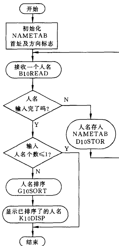
图 6.6 人名排序的程序框图
