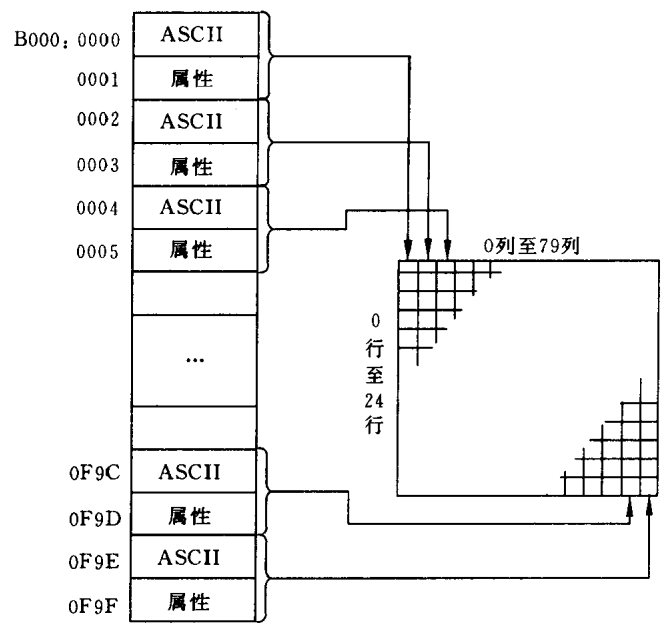
图 9.7 显示存储器单元与显示屏幕上字符对应关系
