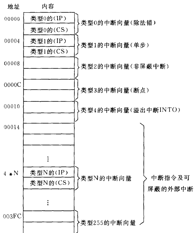
图 3.27 基于 8086 的微机存储器中的中断向量区
