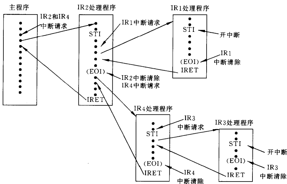
图 8.8 正常优先级方式下的典型中断序列
