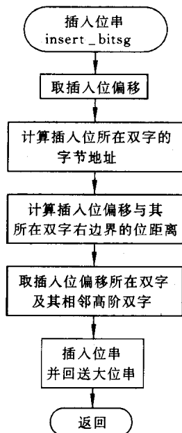
(3) 插入位串子程序框图
