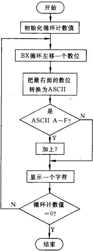
图 5.2 二进制到十六进制数转换的程序框图
