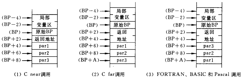
图 6.3 几种高级语言过程调用时的堆栈情况
