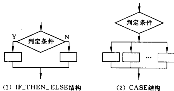
图 5.10 分支程序的结构形式
