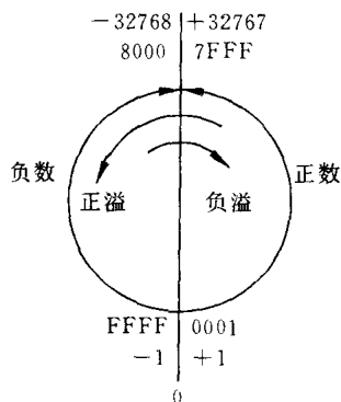
图 3.23 16 位二进制补码表示数的范围
