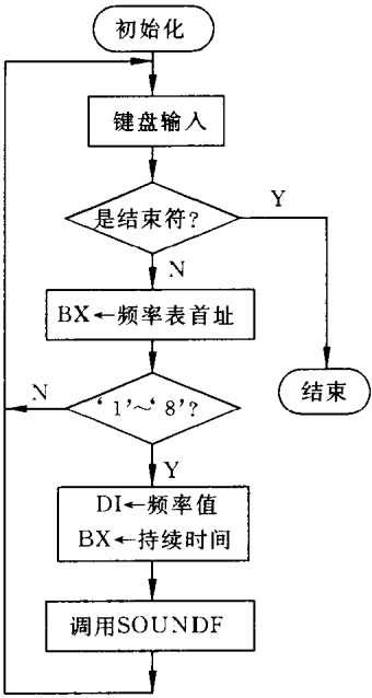
图 10.13 PIANO 程序框图
