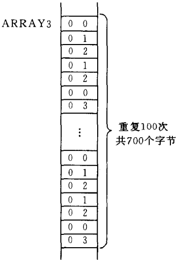
图 4.6 例 4.11 的汇编结果
