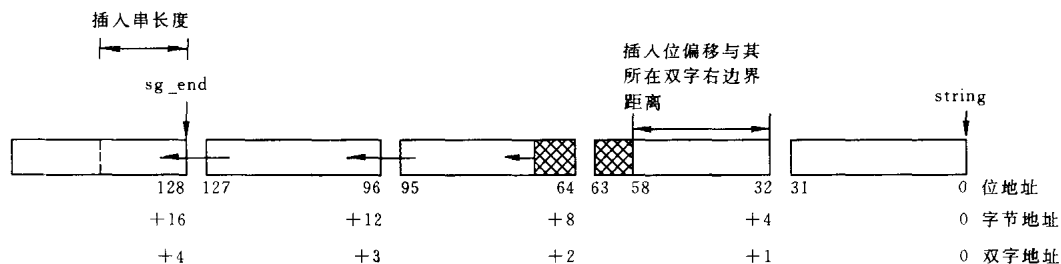
图 6.8 大位串及插入子串举例(位偏移为 58,子串长度为 15 位。)
