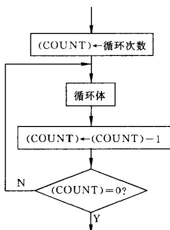
图 3.24 循环程序框图
