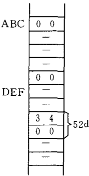
图 4.4 例 4.9 的汇编结果
