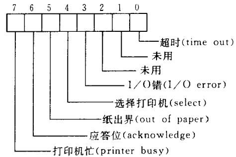
图 9.8 打印机的状态字节
