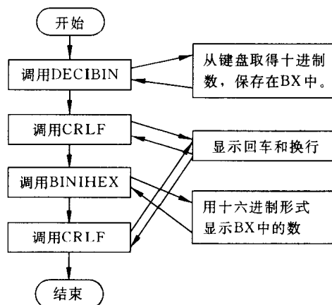
图 6.1 十进制到十六进制数转换的程序结构
