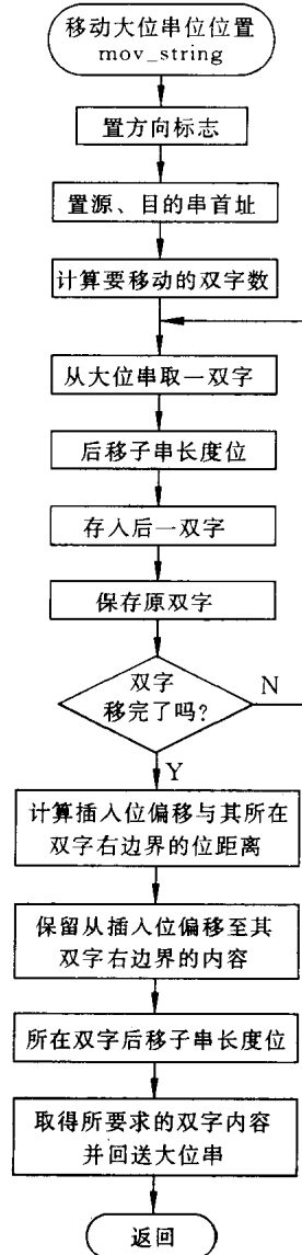
(2) 移动大位串位置子程序框图
