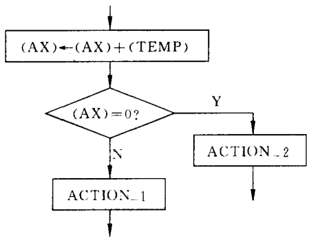
图 3.22 例 3.74 的程序框图
