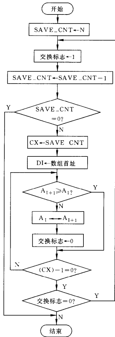
图 5.9 例 5.8 起泡排序算法的程序框图
