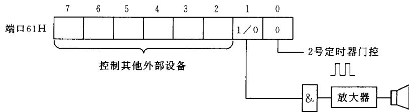
图 8.1 设备控制寄存器
