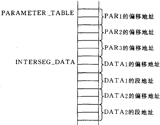
图 4.7 例 4.12 的汇编结果
