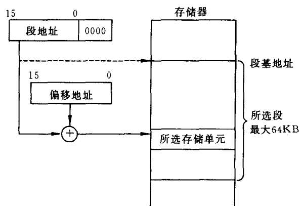
图 2.8 实模式存储器寻址
