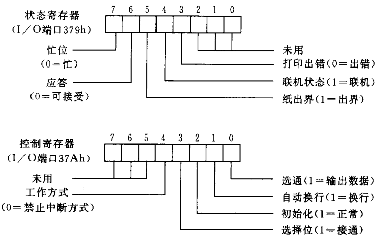
图 8.2 打印机的状态寄存器和控制寄存器
