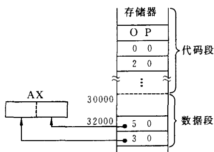
图 3.3 例 3.5 的执行情况
