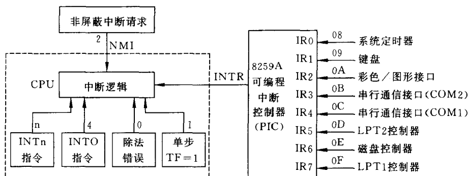
图 8.3 80x86 中断源
