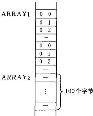
图 4.5 例 4.10 的汇编结果
