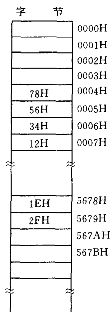
图 2.6 存储单元的地址和内容
