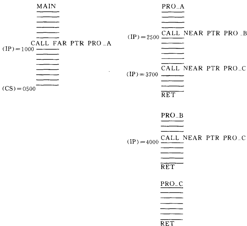
图 3.25 例 3.82 的子程序调用关系
