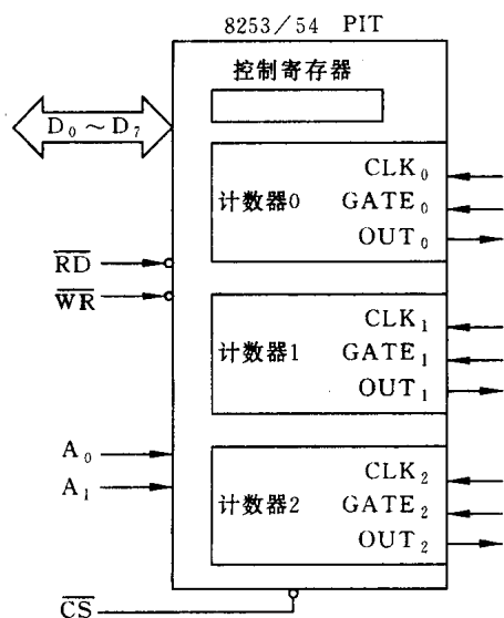
图 10.7 8253/54 的编程结构
