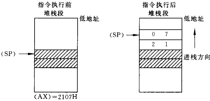
图 3.10 PUSH AX 指令的执行情况
