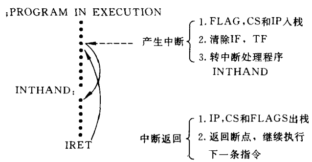
图 8.7 中断过程
