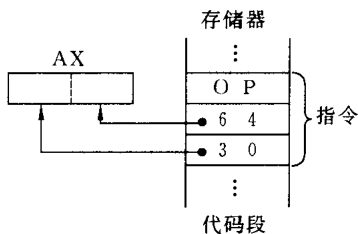
图 3.2 例 3.2 的执行情况
