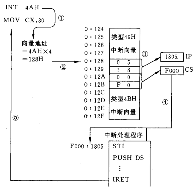
图 8.6 中断操作步骤
