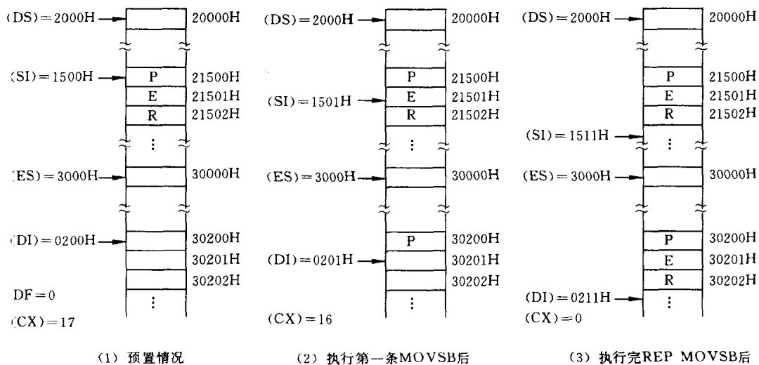
图 3.16 REP MOVSB 指令的执行情况
