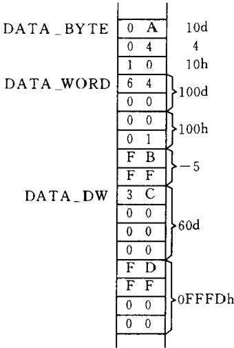
图 4.2 例 4.7 的汇编结果
