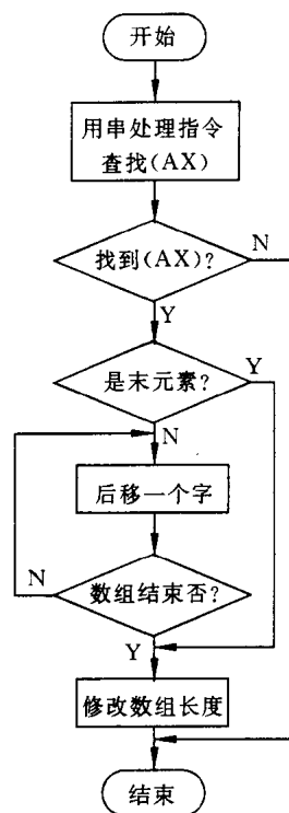
图 5.4 删除数组中一元素的程序框图
