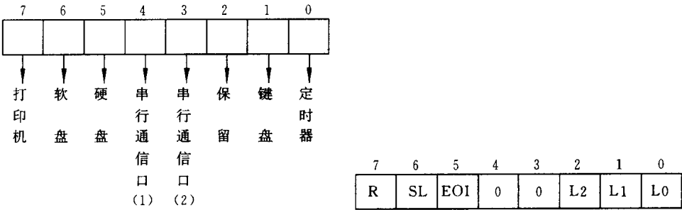
(a) 中断屏蔽寄存器(I/O端口21H) (b) 中断命令寄存器(I/O端口20H)
