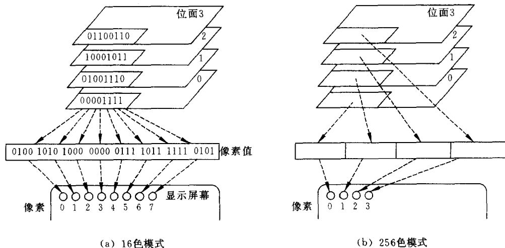
图 10.2 EGA 和 VGA 的位面结构
