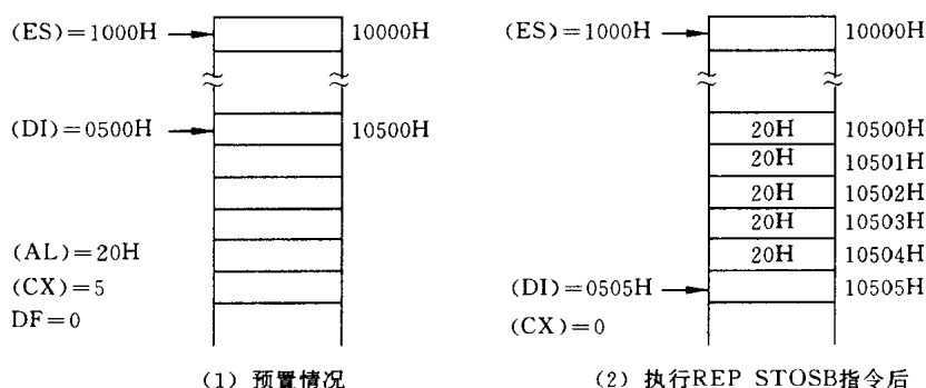
图 3.17 REP STOSB 指令的执行情况
