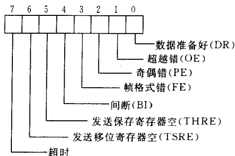
图 9.13 串行通信口状态字节
