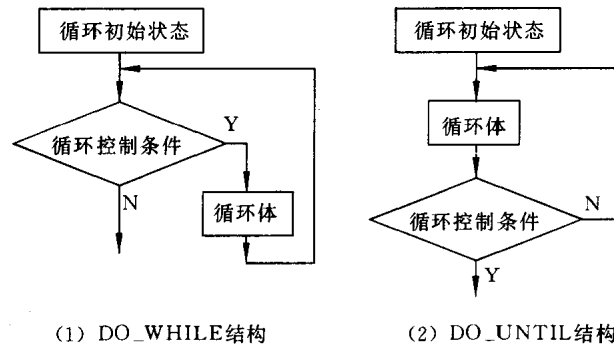
图 5.1 循环程序的结构形式
