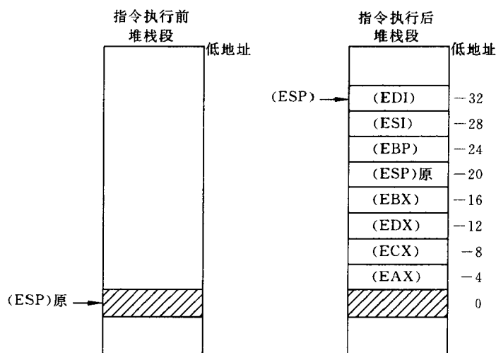
图 3.12 PUSHAD 指令的执行情况
