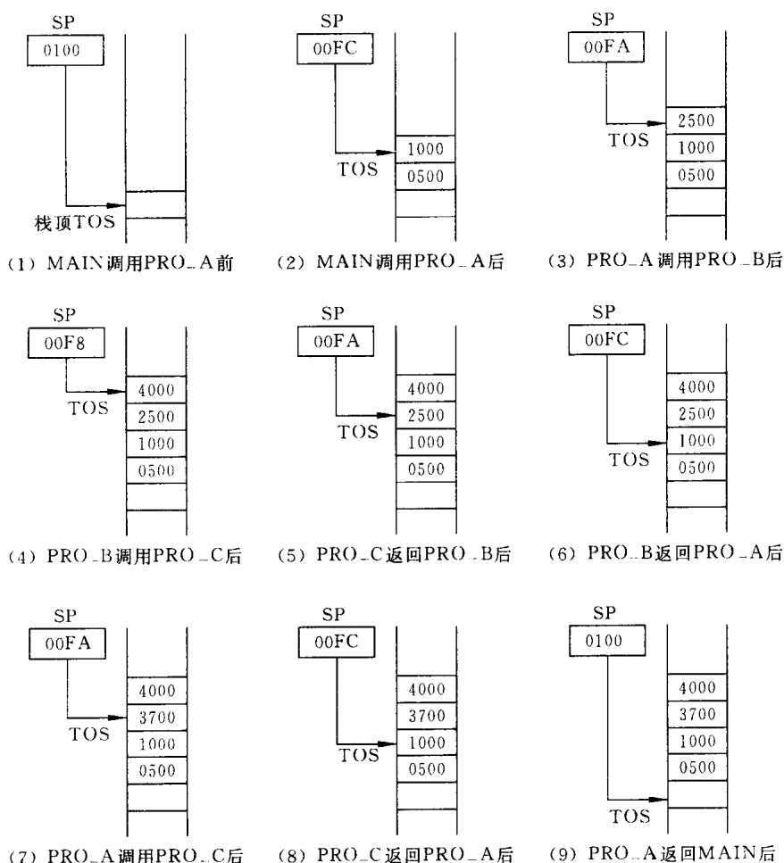
图 3.26 例 3.82 的堆栈情况
