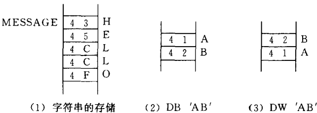
图 4.3 例 4.8 的汇编结果
