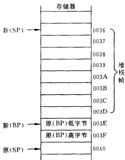
图 3.28 ENTER 8, 0 指令所建立的堆栈帧
