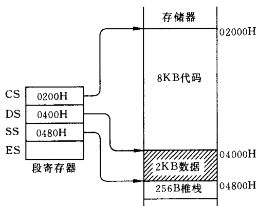
图 2.10 段分配方式之二
