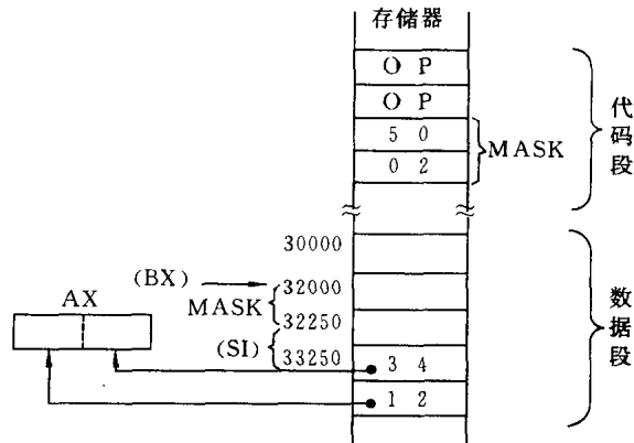
图 3.7 例 3.11 的执行情况
