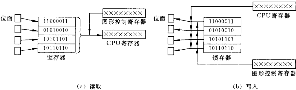
图 10.4 EGA/VGA 图形方式下 CPU 读(a)写(b)时的数据流
