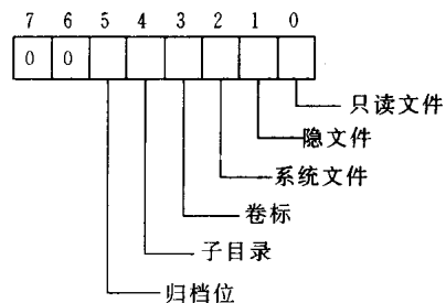
图 11.2 文件属性字节
