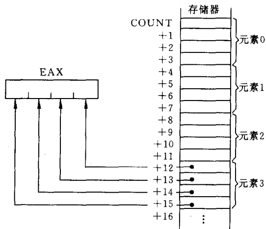
图 3.8 例 3.12 的执行情况
