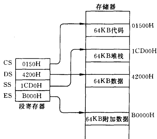
图 2.9 段分配方式之一
