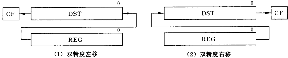
图 3.15 双精度移位指令的操作
